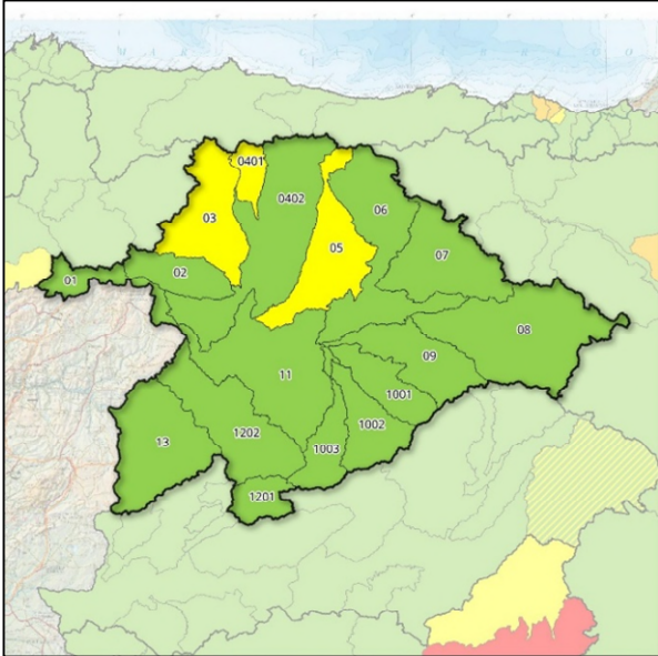
Mapa escenarios escasez por UTE. Agosto 2025
