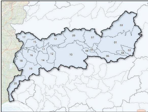
Mapa sequía prolongada por UTS. Agosto 2025
