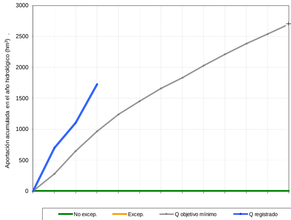
Gráfico 4-2. Aportación mensual acumulada en el salto de Cedillo
