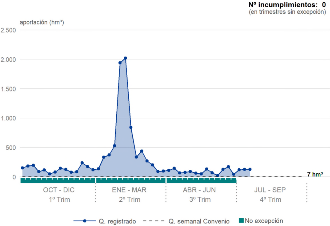
Gráfico 19. Aportación semanal en Cedillo.
