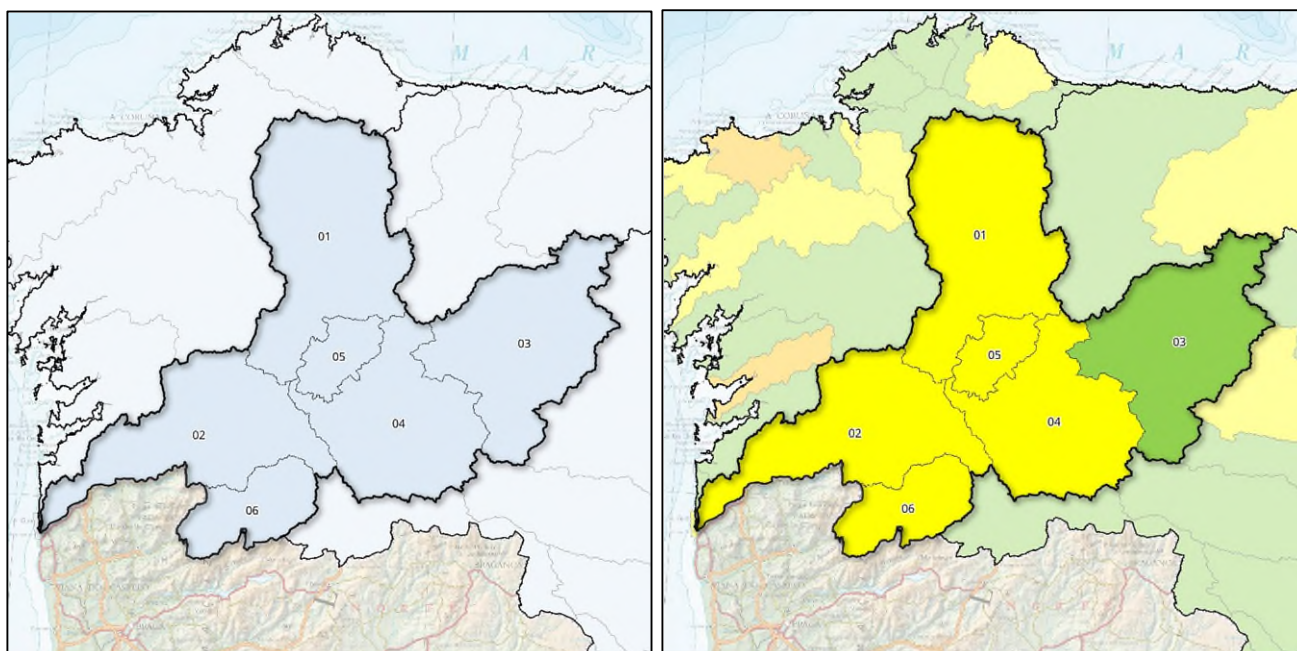
Figura 1. Mapas de sequía prolongada por UTS (izq.) y escenarios escasez por UTE (dcha.). DH Miño-Sil. Julio 2026.
