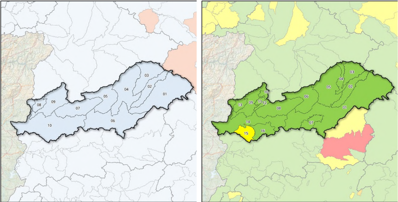
Figura 3. Mapas de sequía prolongada por UTS (izq.) y escenarios escasez por UTE (dcha.). DH Tajo. Julio 2026.
