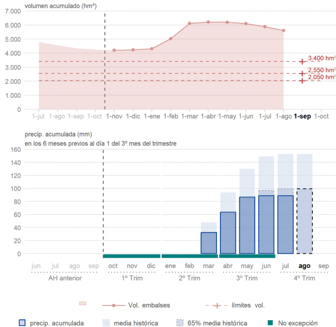
Gráfico 22. Precipitaciones de referencia (Talavera, Ciudad Real) acumuladas en 6 meses hasta el día 1 del tercer mes del trimestre versus valores históricos y volumen acumulado en los embalses de referencia.
