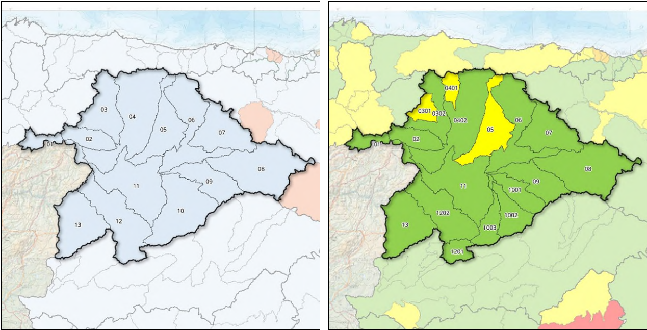
Figura 2. Mapas de sequía prolongada por UTS (izq.) y escenarios escasez por UTE (dcha.), DH Duero. Julio 2026.
