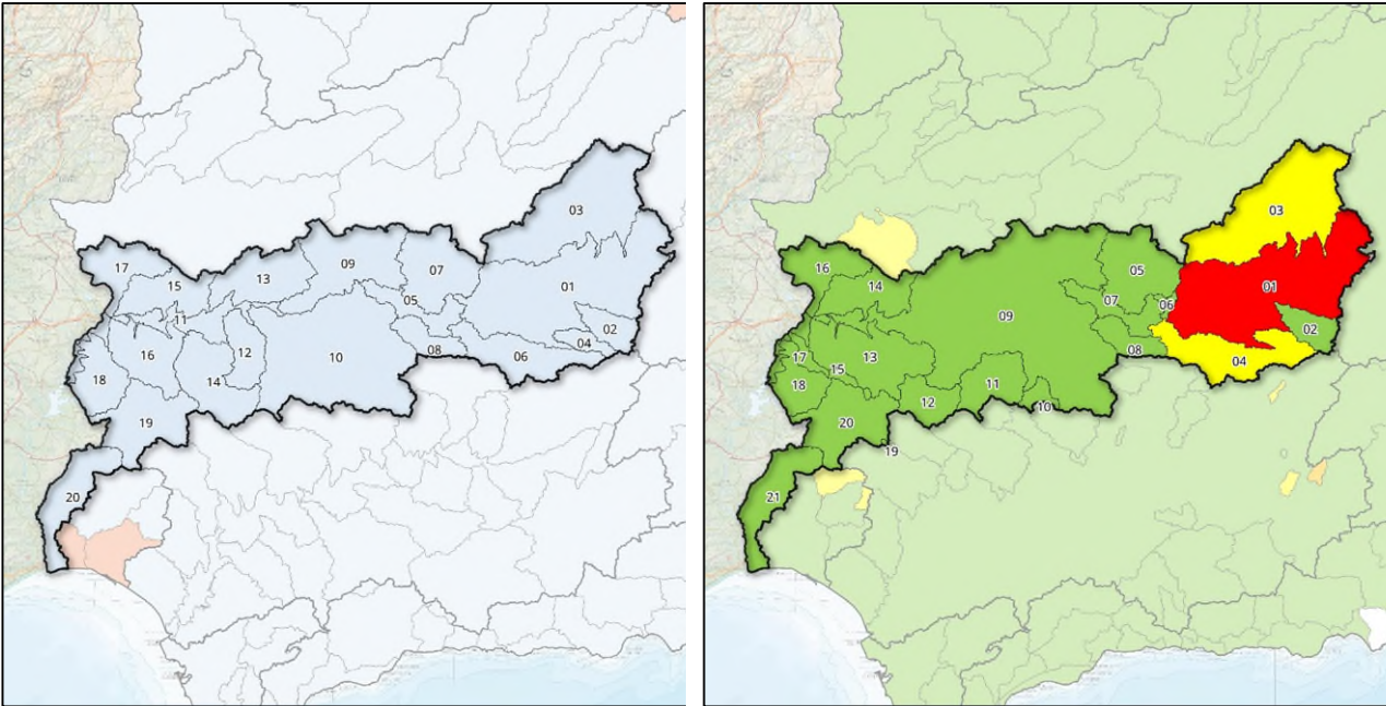
Figura 4. Mapas de sequía prolongada por UTS (izq.) y escenarios escasez por UTE (dcha.), DH Guadiana. Julio 2026.
