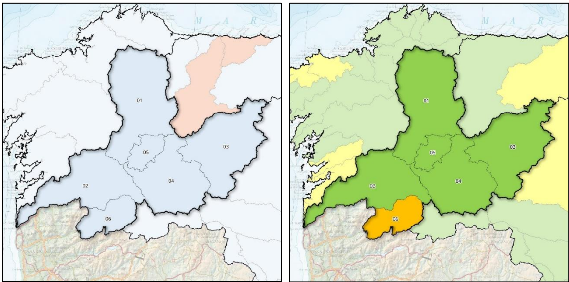
Mapa sequía prolongada por UTS. Septiembre 202 Mapa escenarios escasez por UTE. Septiembre 2025
