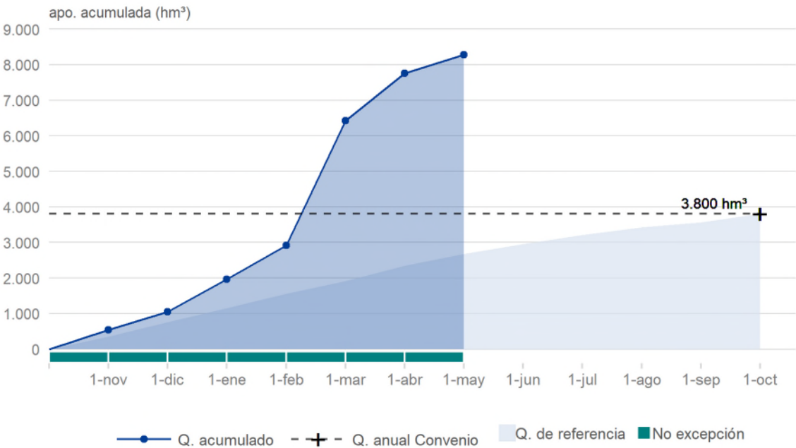
Gráfico 11. Aportación mensual acumulada en Saucelle y río Águeda.
