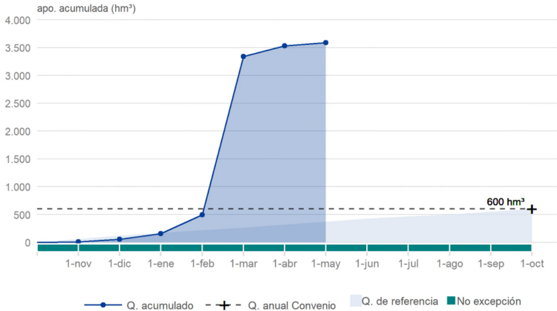
Gráfico 21. Aportación mensual acumulada en el Azud de Badajoz.
