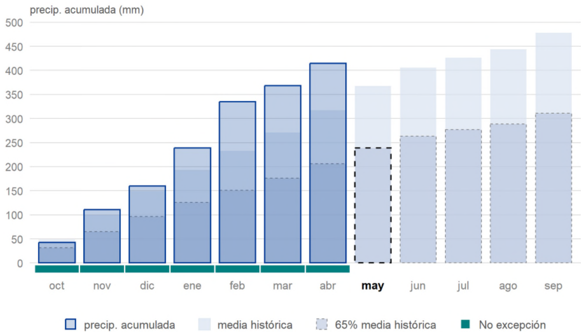
Gráfico 10. Precipitaciones de referencia (Salamanca, Valladolid, León, Soria) en el año hidrológico versus valores histórico.
