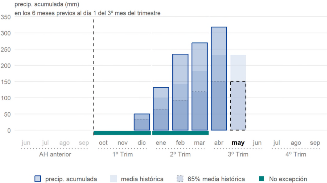
Gráfico 7. Precipitaciones de referencia (Valladolid, León, Soria) acumuladas en 6 meses hasta el día 1 del tercer mes del trimestre versus valores históricos.
