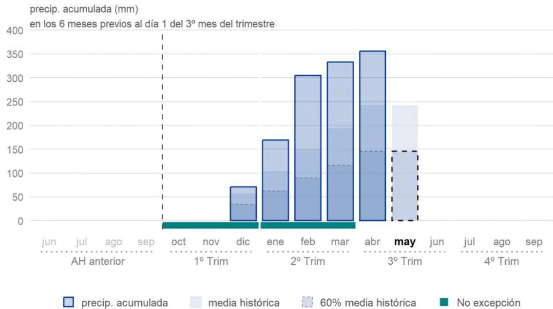
Gráfico 17. Precipitaciones de referencia (Cáceres Madrid) acumuladas en 6 meses hasta el día 1 del tercer mes del trimestre versus valores históricos.
