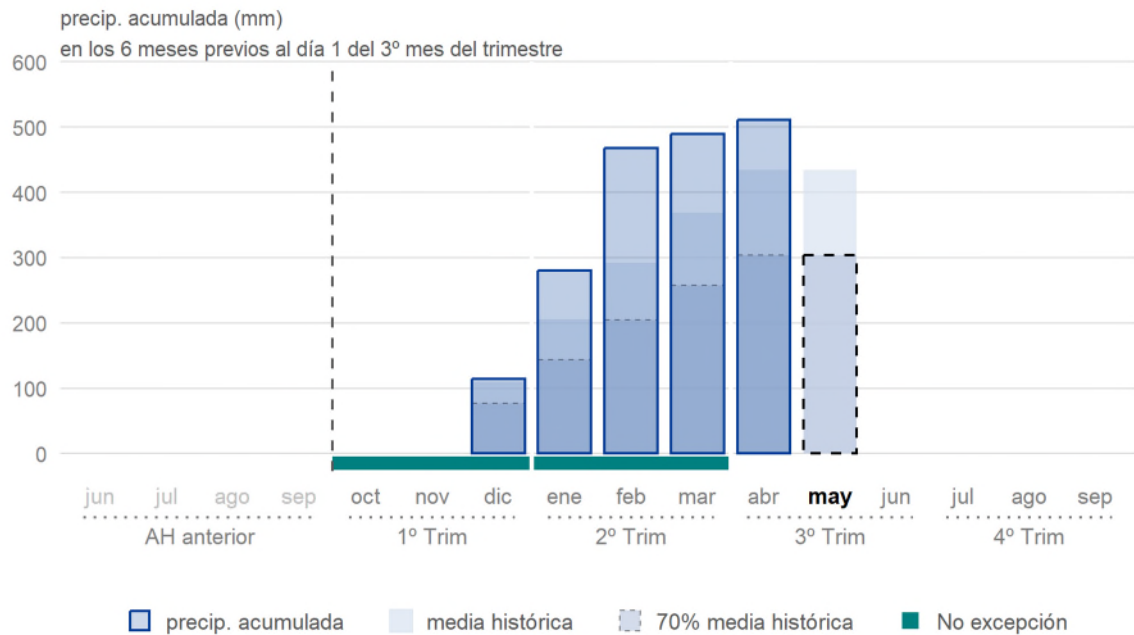
Gráfico 3. Precipitaciones de referencia acumuladas en 6 meses hasta el día 1 del tercer mes del trimestre versus valores históricos (Lugo, Orense, Ponferrada).
